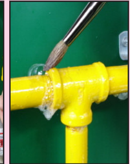
가스배관 연결부위
